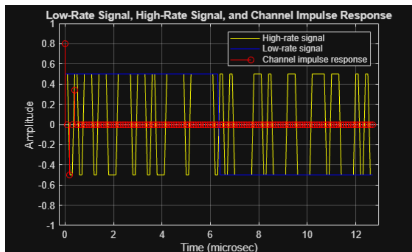
รูปที่ 2.1 (อ้างอิง: Mathworks Introduction to OFDM)
