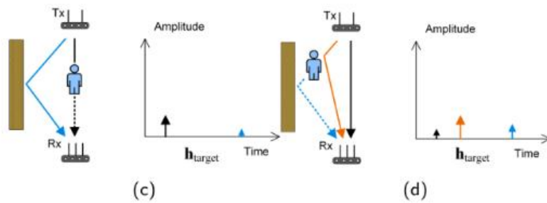
รูปที่ 2.6 (อ้างอิง: Yang et al., 2026, หน้า 3-4, รูปที่ 1(c)-(d))
