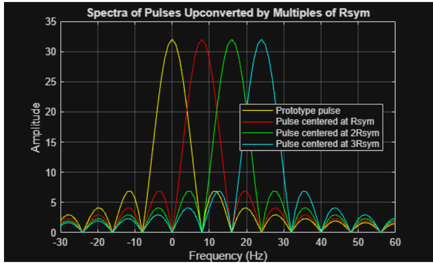
รูปที่ 2.4 (อ้างอิง: Mathworks Introduction to OFDM)
